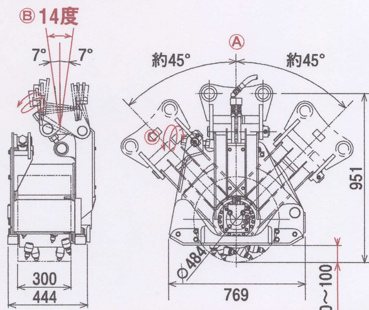
■エスカルゴン 仕様図(mm)
