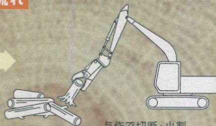
与作で切断・小割
