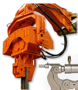
エイパイラー(0.25 m 3 )
